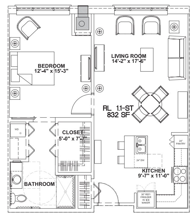
1 RL 1.1 STANDARD SCALE: 1/4"=1'-0"
