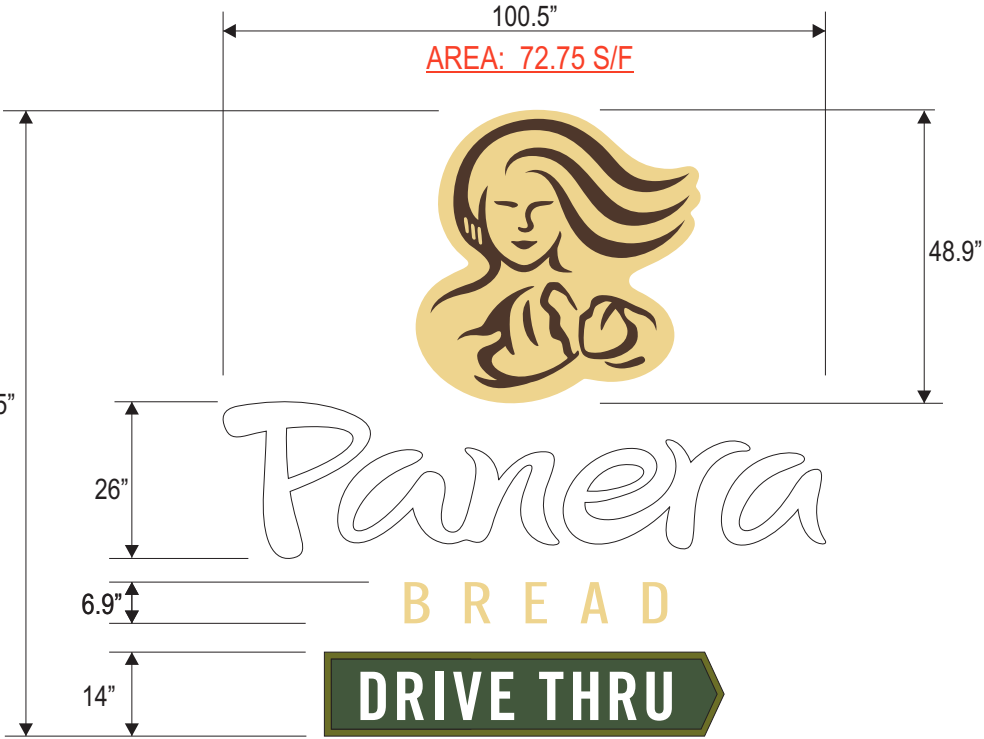
SCALE: 3/8" = 1'-0"
